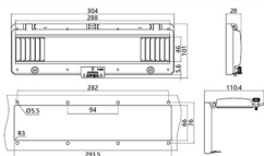
型号 Model SHW-16A (16回路) : 长101×宽304×高28 尺寸图 Dimension drawing
