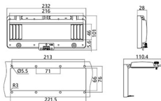
型号 Model SHW-12A (12回路) : 长 101×宽 232×高 28 尺寸图 Dimension drawing
