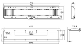
型号 Model SHW-24A (24回路) : 长101×宽448×高28 尺寸图 Dimension drawing
